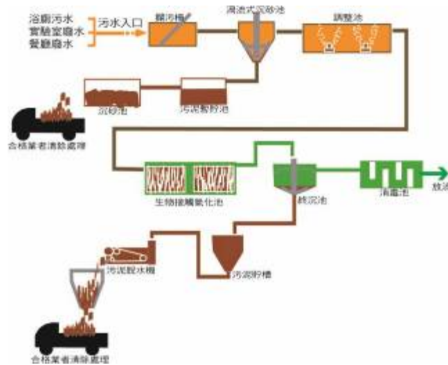
校區廢水處理流程圖
